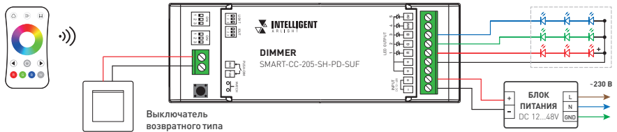
Рис. 3. Схема подключения диммера для управления RGB-нагрузкой
